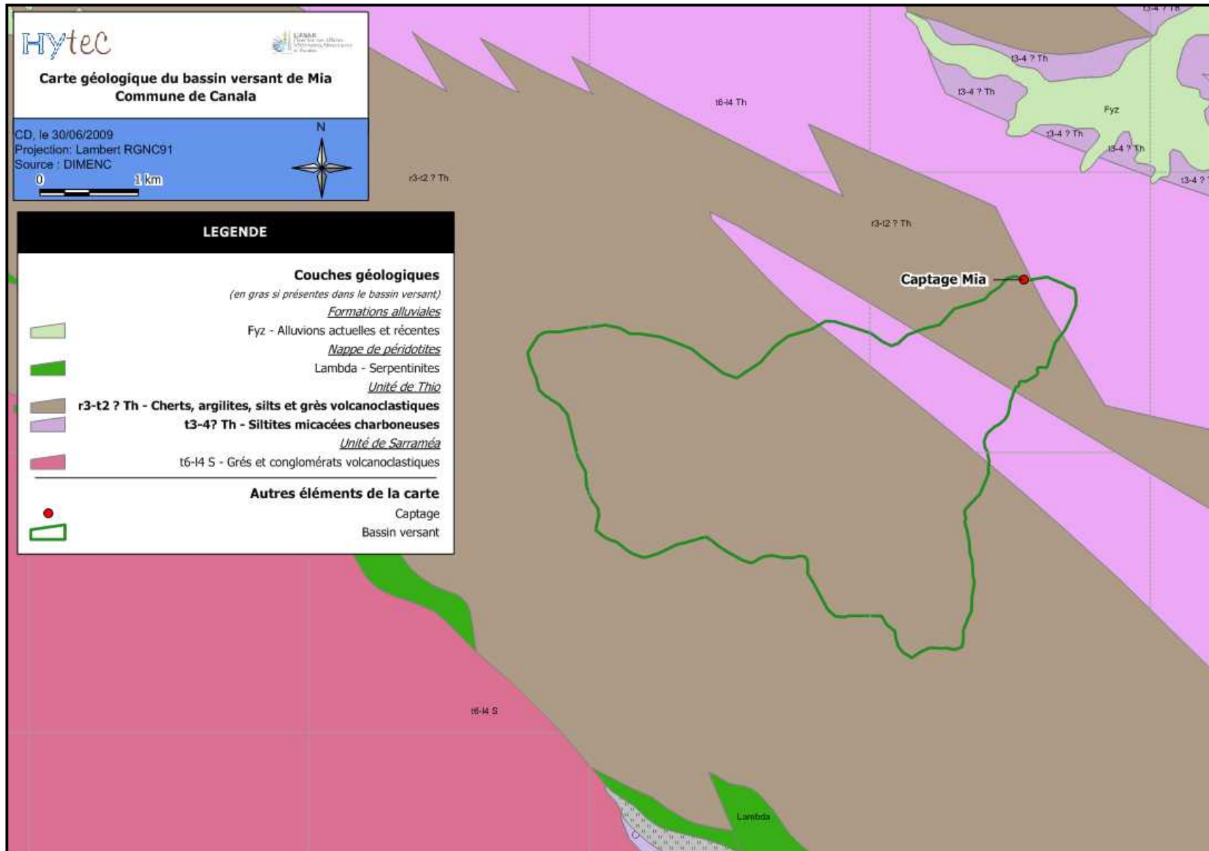
Figure 1 : Représentation cartographique des formations géologiques du bassin versant du captage de Mia Kupe
