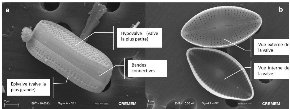
Figure 1 : Frustule de Nitzschia amphibia (a) ; Frustule ouvert de Diadesmis confervacea (b) (microscopie électronique à balayage).
