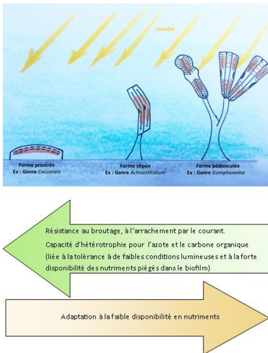
Figure 3 : Facteurs environnementaux structurant les communautés de diatomées.
